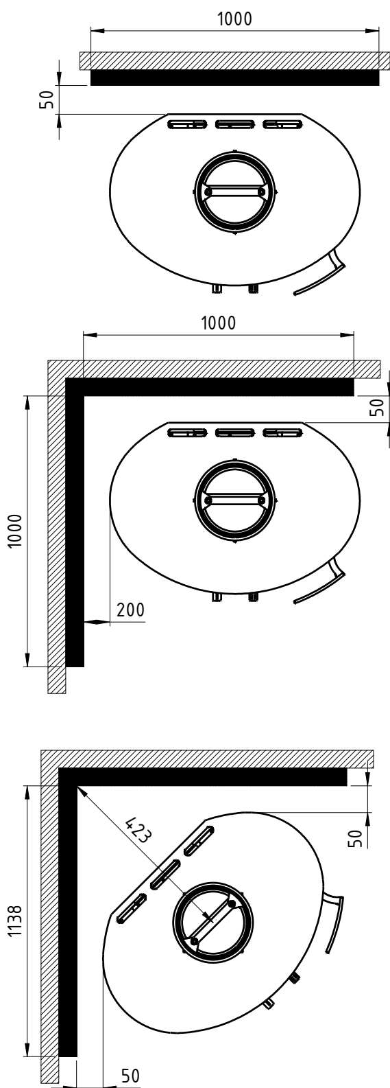
Ild 9 ECO and 11 ECO - senza vetro laterale
